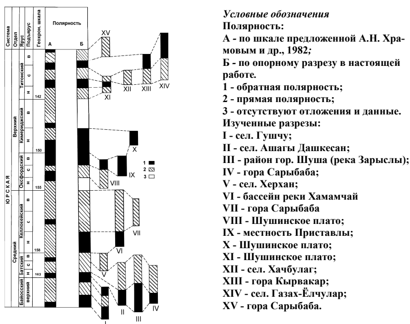
Рис. 1. Палеомагнитная шкала средней и верхней юры по магнитостратиграфическим данным Малого Кавказа (Азербайджан).
